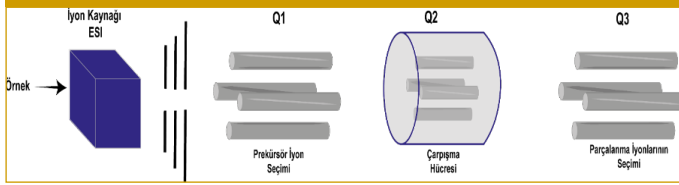
Şekil 6.15. MS/MS Sistemi
